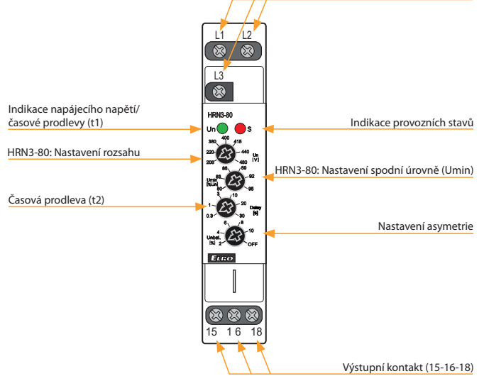
Svorky napájecí/hlídaného napětí (L1-L2-L3)
