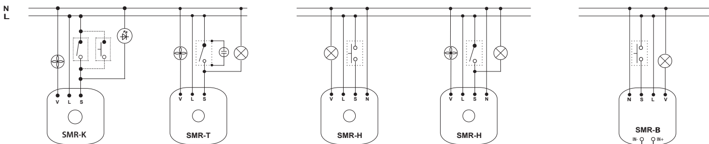
Typické zapojení SMR-K, - časovač pro ventilátor
