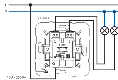
VYPÍNAČ DVOUPÓLOVÝ, OVLÁDANÝ TAHEM (ŠŤŮRKOU)
