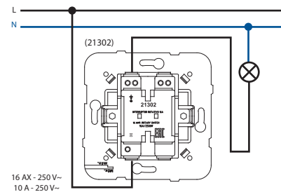
OTOČNÝ PŘEPÍNAČ 16 A TLAČÍTKO OVLÁDANÉ TAHEM 10 A
